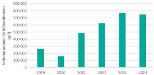
Graphique 4 — Evolution du volume annuel de débordement aux réservoirs de Pontacq
